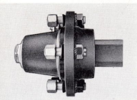
Smitt hjulnav med stefatning av fabrikat PML samt 60 mm axel av specialstål.
