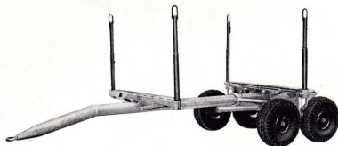
ROTTNE 6 TON BOGGI best.-nr 462
