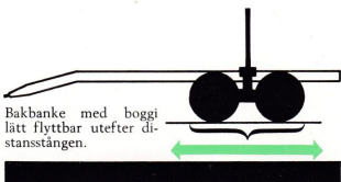
Triangelstjadgad boggi, helt okänslig för vridpåkänningar vid svängar. Boggiaxeln placerad bakom centrum för lättare hindertagning.
