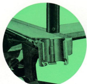
Rottne 6 och 8 ton boggi har bankar med bottenutlösning, som utlöses från motsatt sida. Extra säkring mot ofrivillig utlösning.
